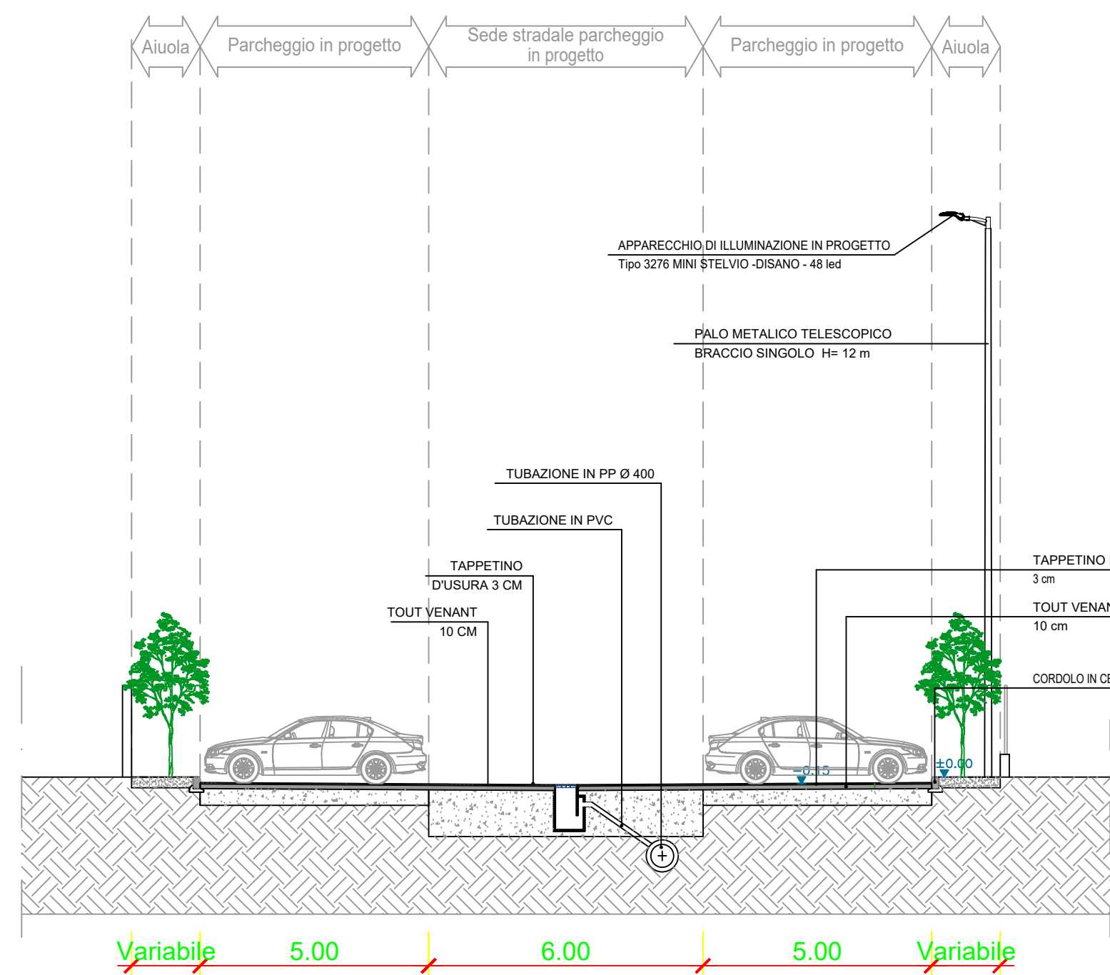
STATO DI PROGETTO - SEZIONE A-A Scala 1:100
