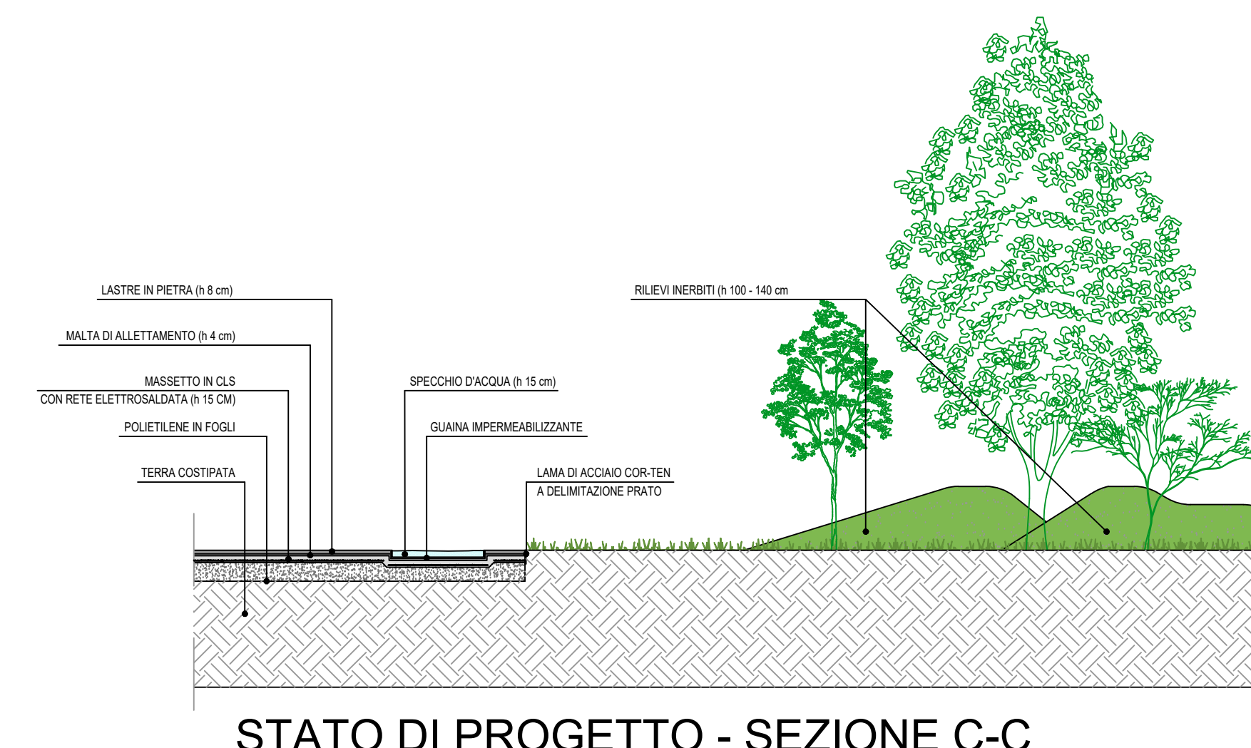
STATO DI PROGETTO - SEZIONE C-C Scala 1:100
