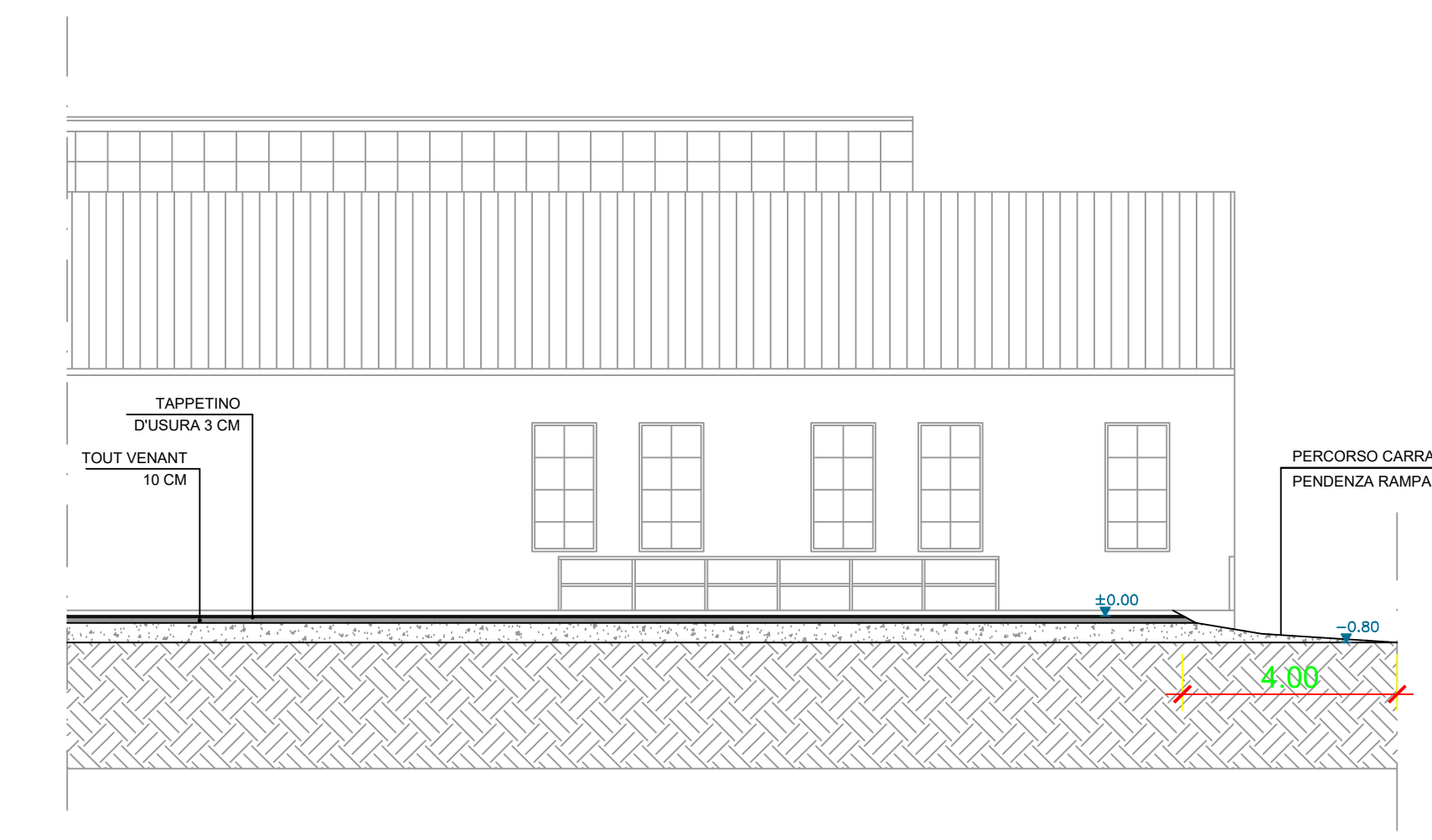
STATO DI PROGETTO - SEZIONE D-D Scala 1:100
