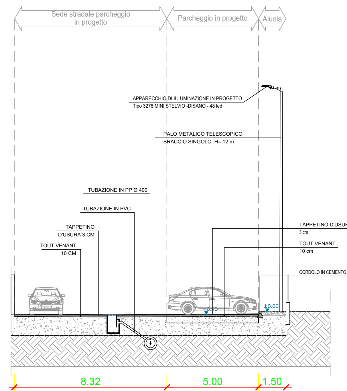
STATO DI PROGETTO - SEZIONE B-B Scala 1:100
